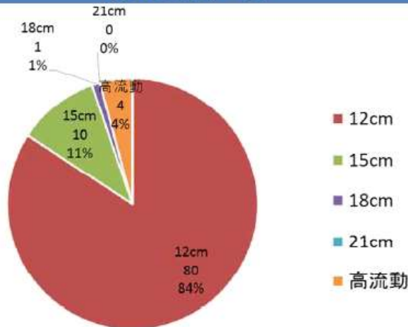
材料分離抵抗性確認方法 (スランプ値が12cmを超えたもの)
